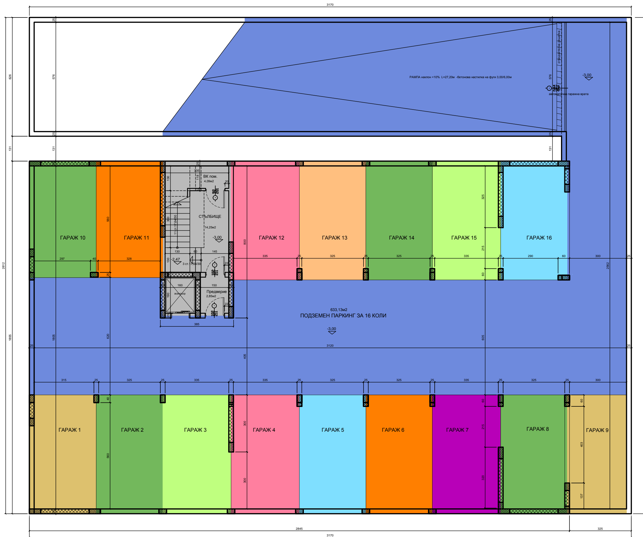
БЛОК "Д" РАЗПРЕДЕЛЕНИЕ СУТЕРЕН
