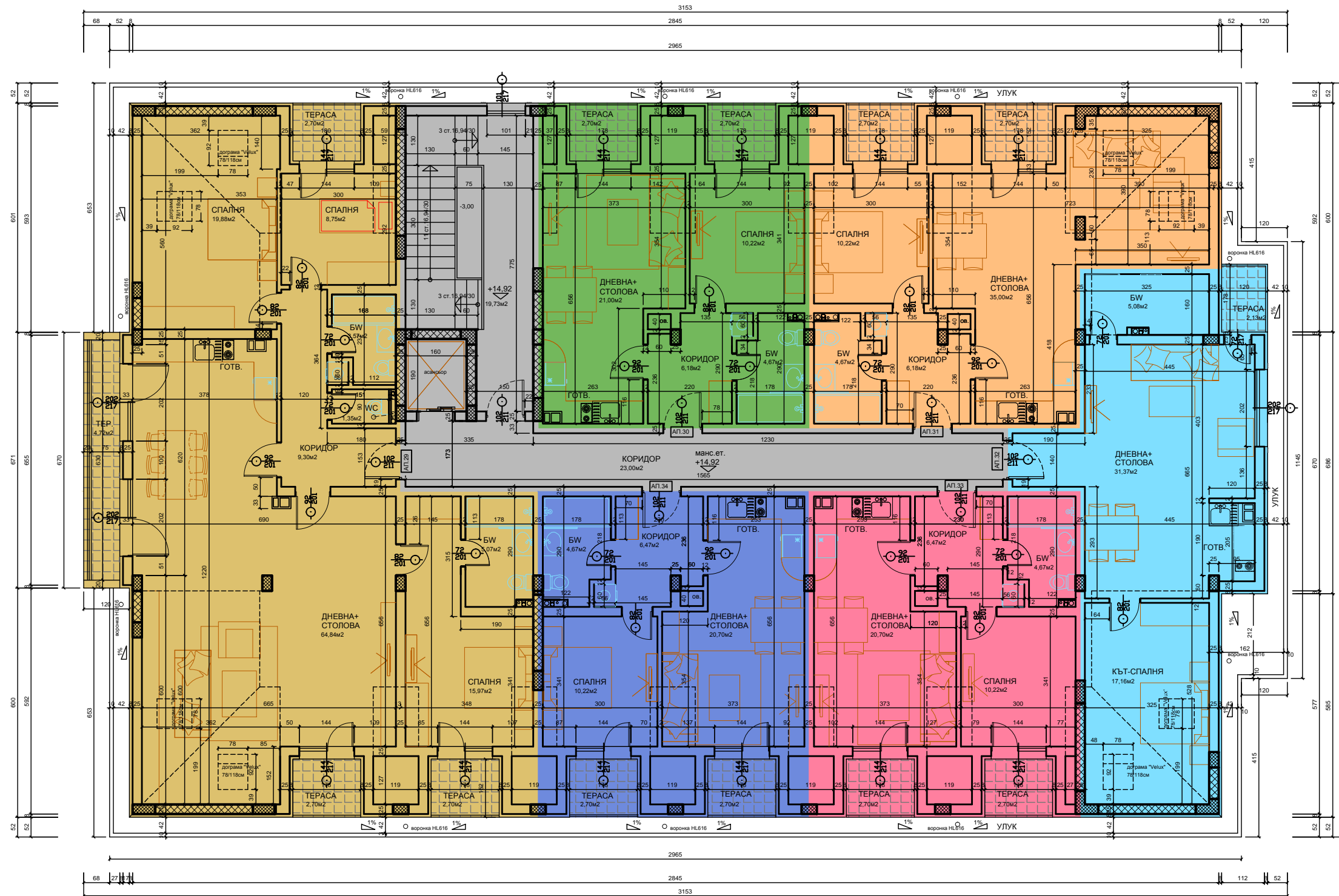
БЛОК "Д" РАЗПРЕДЕЛЕНИЕ МАНСАРДЕН ЕТАЖ
