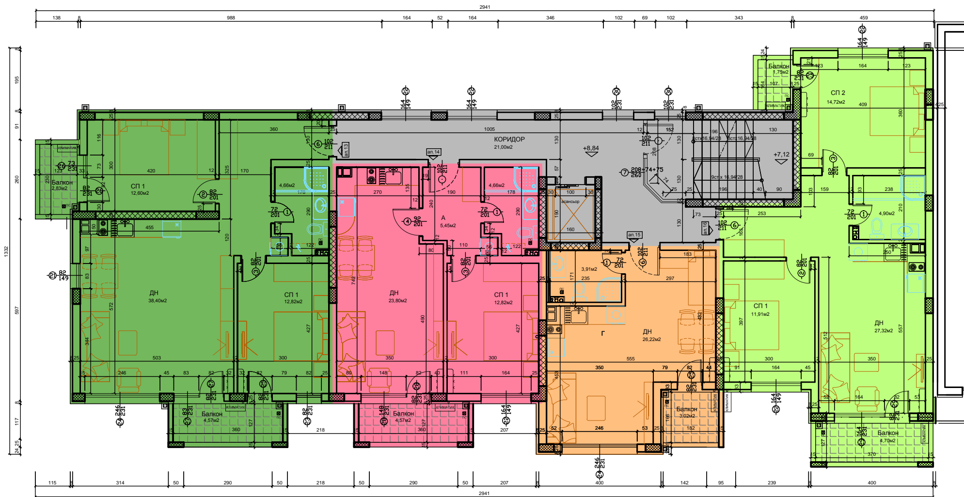
БЛОК "В" РАЗПРЕДЕЛЕНИЕ ЧЕТВЪРТИ ЕТАЖ
