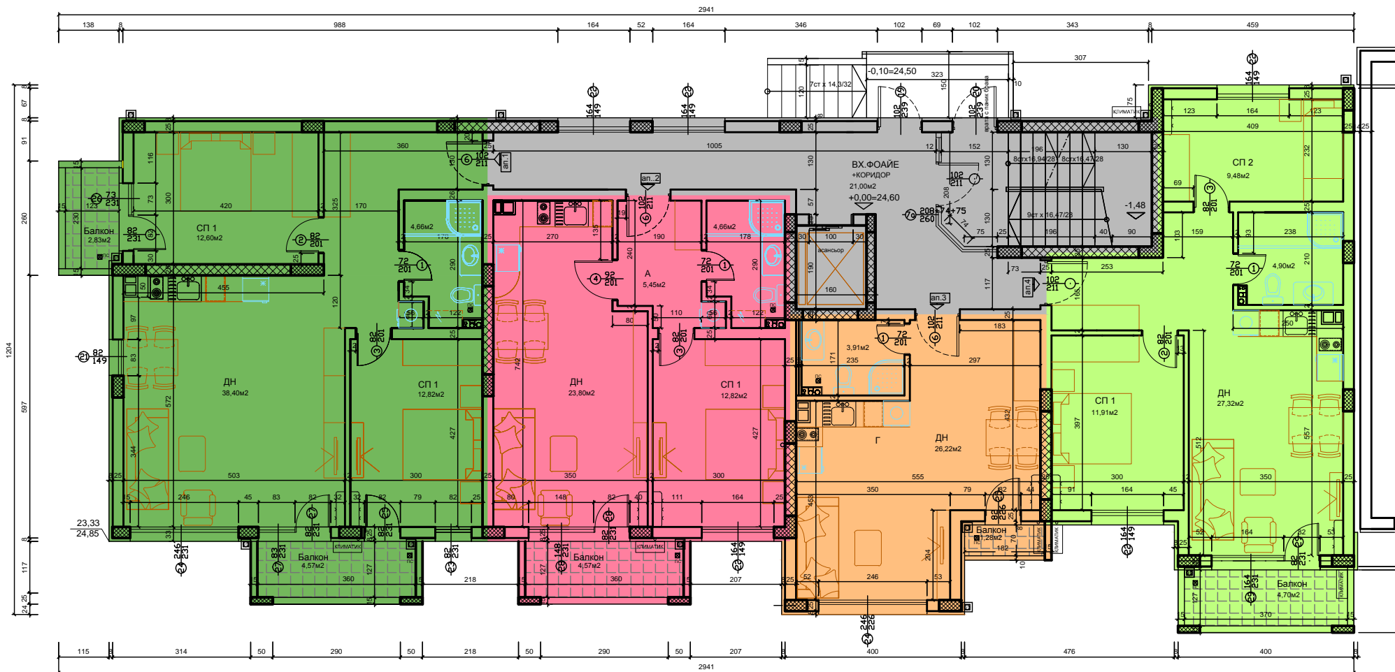
БЛОК "В" РАЗПРЕДЕЛЕНИЕ ПЪРВИ ЕТАЖ
