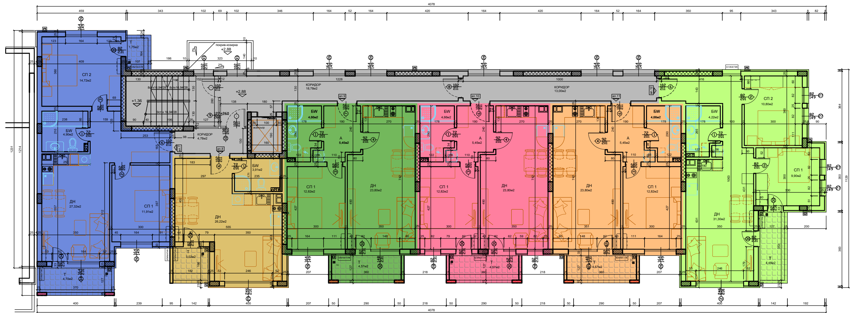
БЛОК "Б" РАЗПРЕДЕЛЕНИЕ ВТОРИ ЕТАЖ
