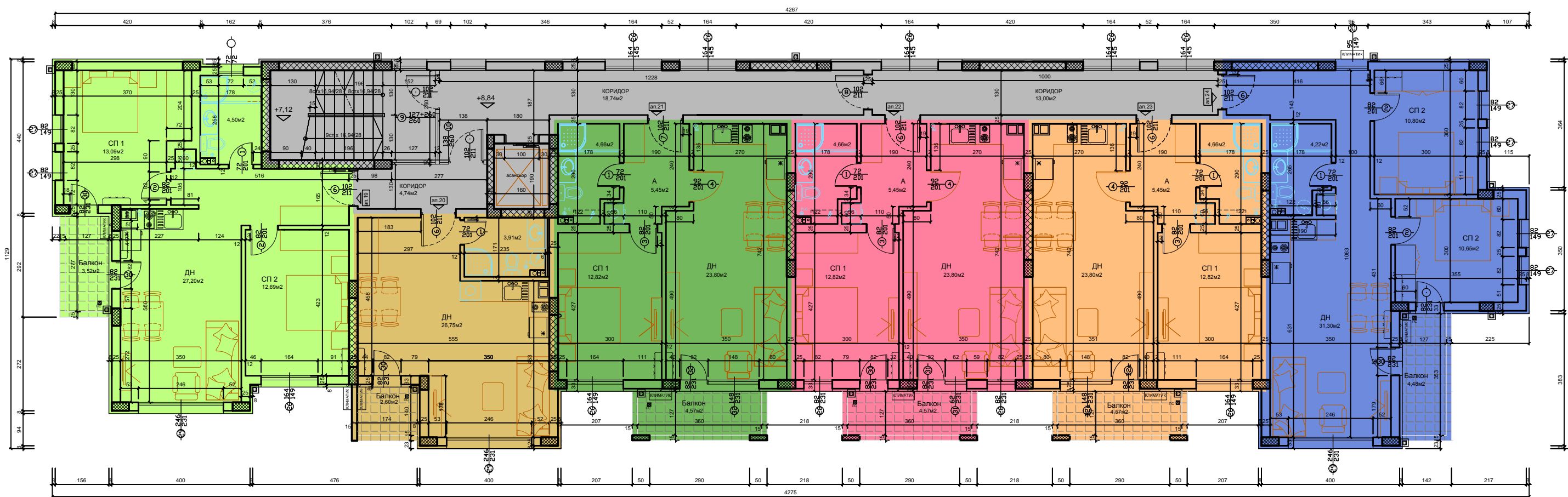
БЛОК "А" РАЗПРЕДЕЛЕНИЕ ЧЕТВЪРТИ ЕТАЖ
